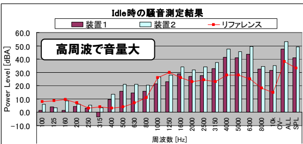
1/3Oct.Band 騒音測定結果
