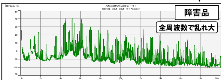
FFT 騒音測定
