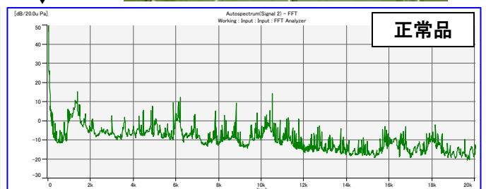
FFT 騒音測定
